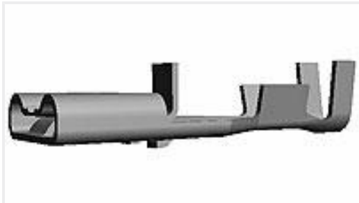
TE 产品编号170329-1 250 PL MKII REC. 15-10AWG PTBR
