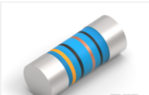
TE 产品编号2176316-9 MELF SMA_A 470R 0.1% 15PPM 0207 1W
