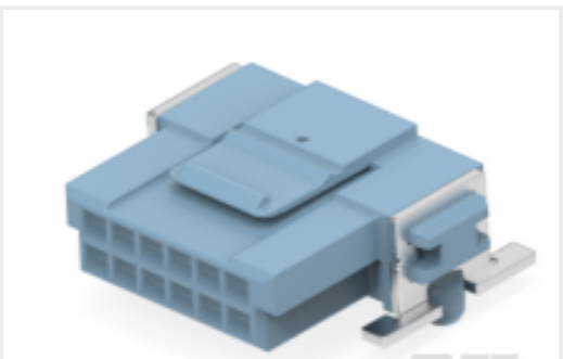
TE 产品编号254262-E SMCQ 12 F AB VV 7-03 CL * 0007 137 E002
