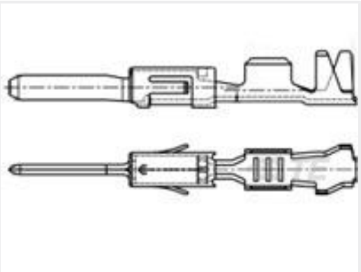
TE 产品编号963904-1 TAB A 1.6x0.6 CONTACT CS SWS Sn
