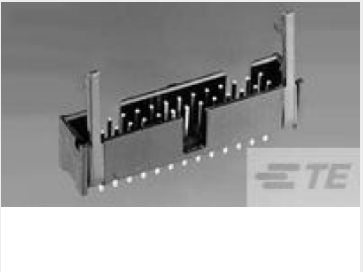
TE 产品编号 2-1761609-8 IDC LOW PRO HDR 24P RA SHT LAT
