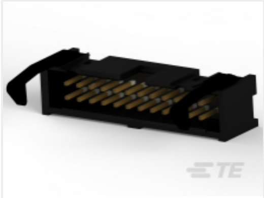
TE 产品编号 1761606-8 IDC LOW PRO HDR 24P VERT LA
