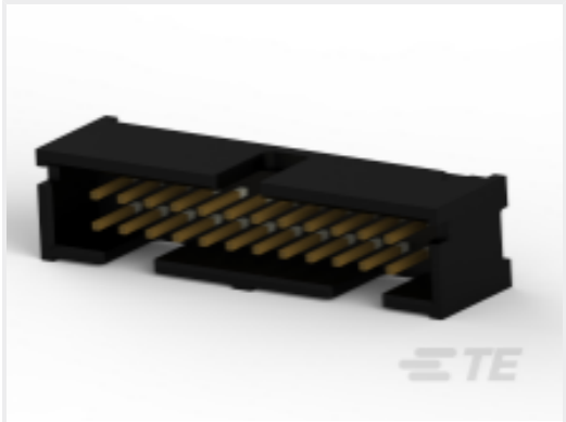
TE 产品编号 1-5103308-3 A/L LOW PRO HDR 24P VERT BLACK
