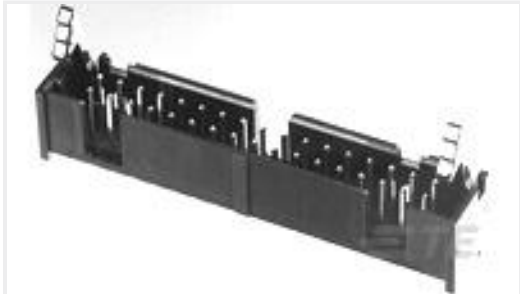
TE 产品编号1-499252-2 030 STRAIN RELIEF A-L RCPT
