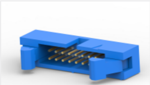
TE 产品编号 1761685-6 IDC LOW PRO HDR 16P VERT SHT LAT
