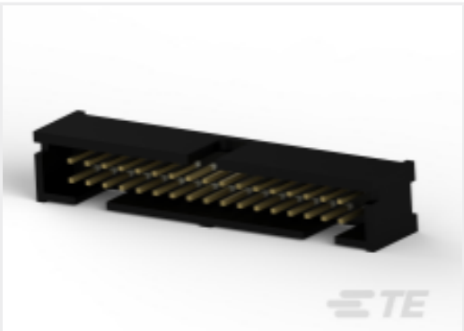
TE 产品编号 5103309-7 A/L LOW PRO HDR 34P VERT BLACK
