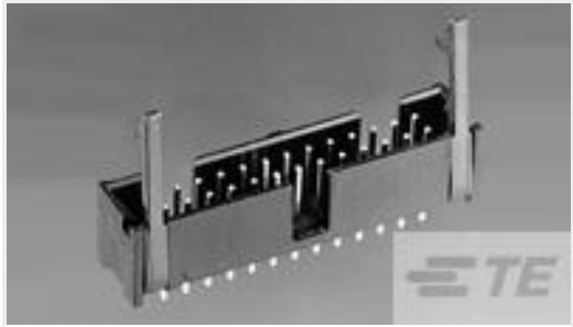
TE 产品编号 2-1761714-6 IDC LOW PRO HDR 16P RA SHT LAT
