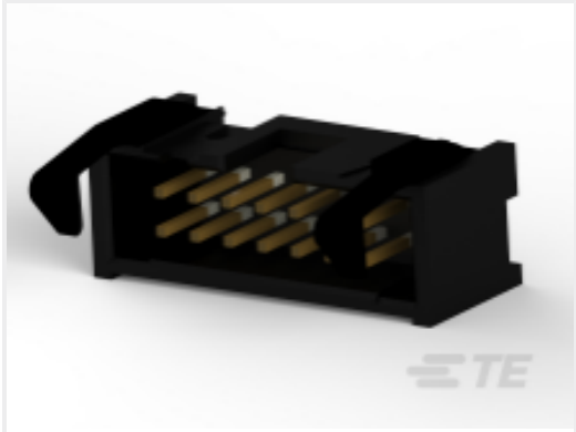
TE 产品编号 1761608-5 IDC LOW PRO HDR 14P VERT SHT L
