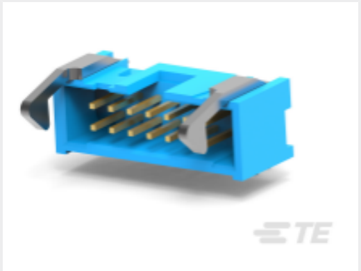
TE 产品编号 2-1761609-5 IDC LOW PRO HDR 14P RA SHT LAT BLUE
