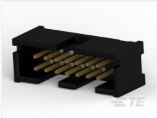
TE 产品编号 5103308-2 A/L LOW PRO HDR 14P VERT BLACK
