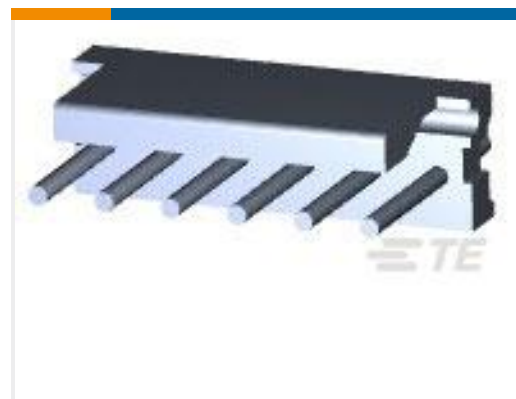
TE 产品编号 640388-6 06P MTA156 HDR ASSY RN STR F/L
