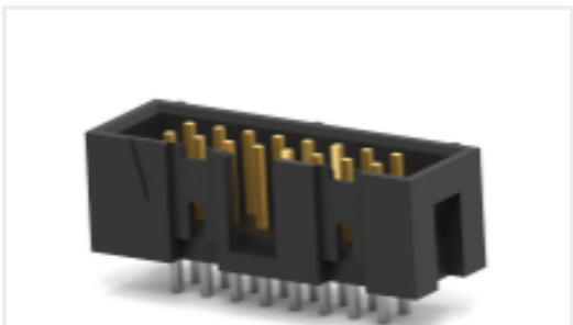
TE 产品编号 1761681-6 IDC LOW PRO HDR 16P VERT HT BLACK
