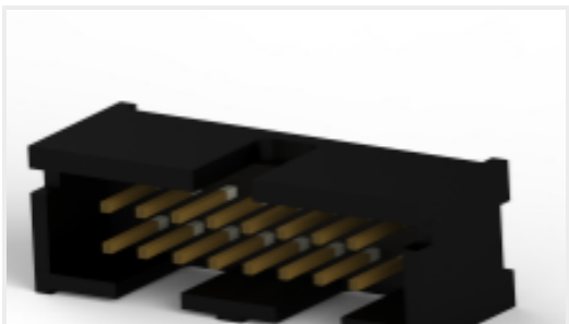
TE 产品编号 5103309-3 A/L LOW PRO HDR 16P VERT BLACK
