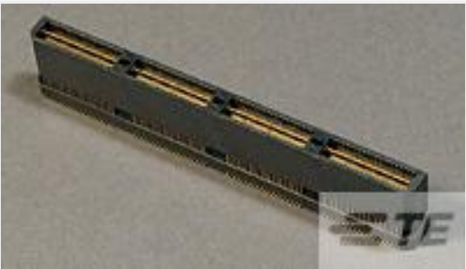
TE 产品编号 2-1658466-4 MSB0.80PL16ASY160FL,-,30,-TY
