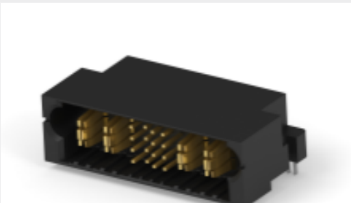
TE 产品编号1-2204910-0 MBXL R/A HDR 2P + 16S + 2P
