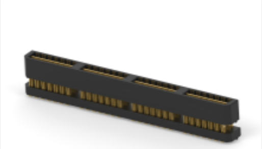
TE 产品编号 1658438-4 MSB0.80PL14ASY160FL,-,10,-TY
