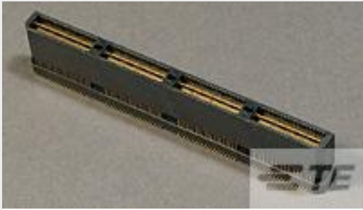
TE 产品编号 1658047-4 MSB0.80PL16ASY160FL,-,F,-TY
