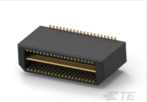
TE 产品编号 6-1658015-1 MSB0.80PL11ASY040FL,GP,10,-TR
