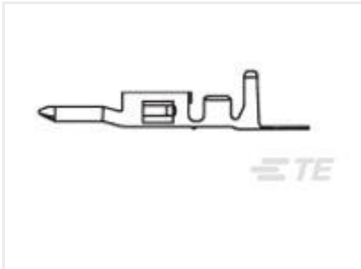
TE 产品编号1586314-2 VAL-U-LOK PIN BR AU 22-18 LP
