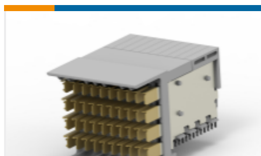
TE 产品编号 6469183-1 HMZD 3PR RA HDR 60P ASSY LF
