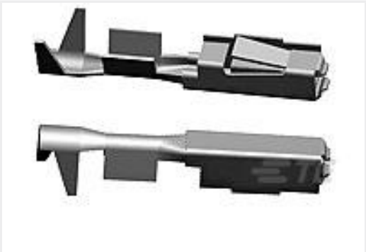
TE 产品编号5-928999-5 MQS0,63 Au rec LL unseal. >0,2-0,35
