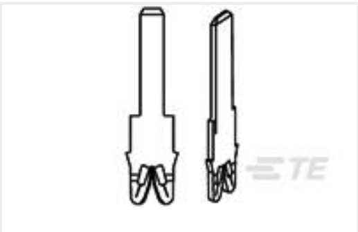
TE 产品编号4-1601090-2 031-161-002=TAB,2.0X.51,STDSMZ
