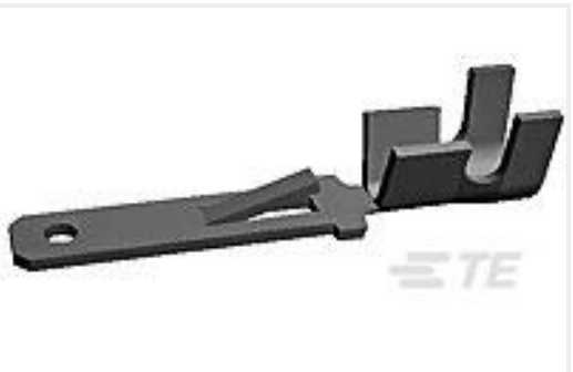
TE 产品编号170058-2 FF 110 TAB 24-20AWG TPBR
