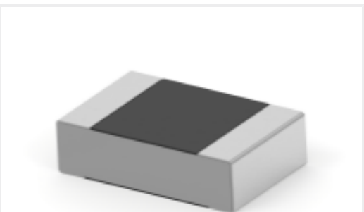
TE 产品编号1-2176264-7 RN 0805 750K 0.1% 10PPM 1K RL
