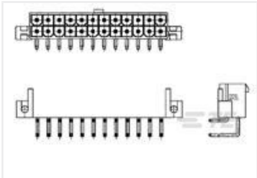
TE 产品编号1-1586043-6 16P VAL-U-LOK R/A HDR SCRMT V2
