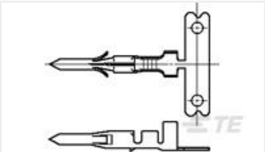
TE 产品编号350629-1 .062 COMM P&S PIN 18-24 PTPBR
