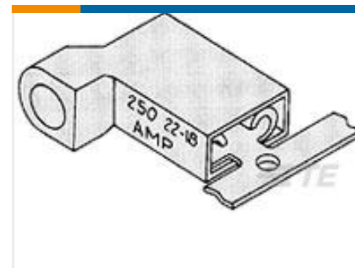
TE 产品编号3-520133-2 ULTRA-FAST 250 ASY REC 16-14 AWG TPBR
