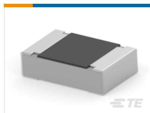
TE 产品编号1-2176342-6 CRGCQ 0805 330R 5%
