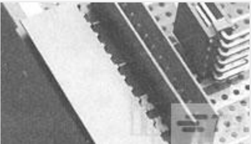
TE 产品编号1-281698-0 HEADER HE14 RA 10 P
