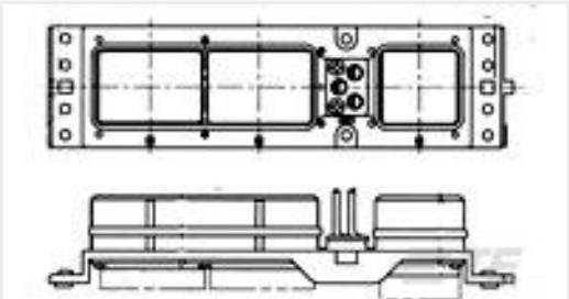
TE 产品编号299147-000 55PC0711-20-4CS2502
