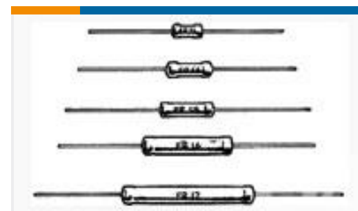
TE 产品编号1623750-6 ER58 15K 5% AMMO
