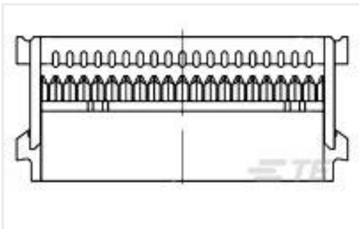
TE 产品编号1658526-4 609-1030LF FEM SOCKT,LEAD FREE
