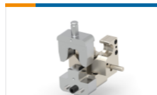
TE 产品编号2234184-1 DIE SET DIA 12MM-90 RIGHT T 50-70MM2
