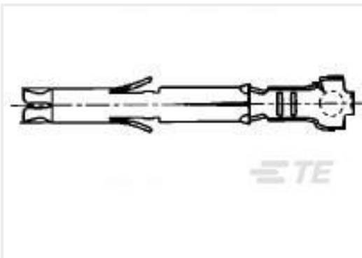
TE 产品编号170365-1 MINI UNIVERSAL M-N-L SOCKET LP
