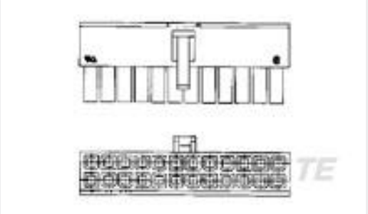
TE 产品编号1586019-8 8P RCPT VAL-U-LOK V0
