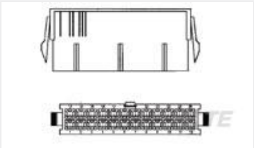
TE 产品编号794953-8 8P PM PLUG VAL-U-LOK V2
