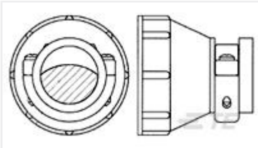
TE 产品编号182658-1 11 SIZE CPC STD CLAMP
