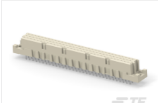
TE 产品编号254897-E STVC 96 F ABC VVV 7-00 TL 4,0 * 137 E007
