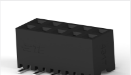
TE 产品编号1-2314846-0 10P,2MM,BB,REC,DRVT,SMD,AU.76, TB,W/CP
