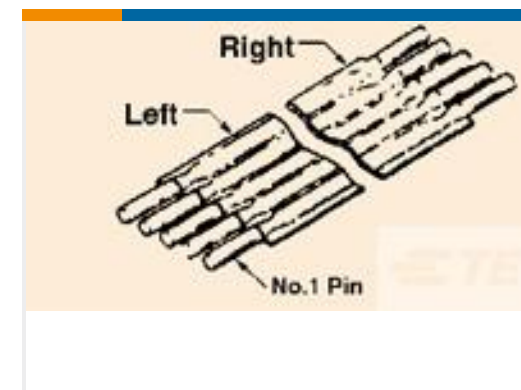
TE 产品编号1437140-9 FSN-21A-4=NOMEX FS STD
