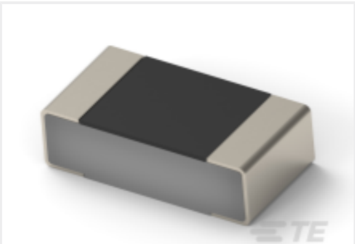
TE 产品编号1879808-6 RP 1J 37R4 0.1% 15PPM 1K RL
