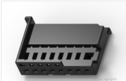
TE 产品编号1394139-1 8POS MQS REC
