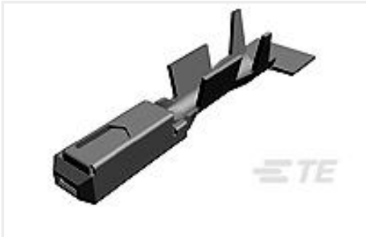
TE 产品编号5-1241608-1 MQS1,5 Sn rec CB unseal. 0,75-1,5
