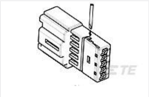
TE 产品编号1-1418778-1 5POS MQS TAB
