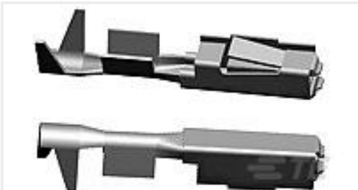
TE 产品编号5-968221-6 MQS0, 63 Ag rec CB unseal. 0,5-0,75
