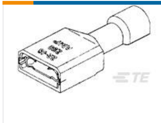
TE 产品编号3-520404-2 ULTRA-FAST 187 ASY REC 16-14 AWG TPBR
