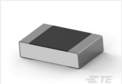
TE 产品编号4-2176374-5 RQ 0805 309R 0.1% 10PPM 1K RL
