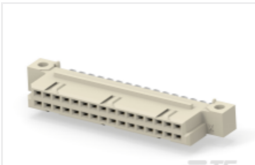
TE 产品编号294722-E STVO/2 32 FI AB VV 7-03 TL * * 247 E 172
