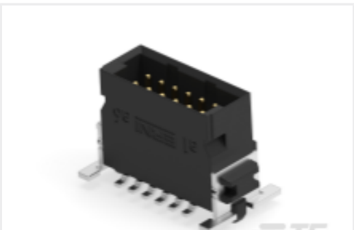
TE 产品编号244854-E SMCQ 12 M AB VV 8-03 CL * H007 137 E005
