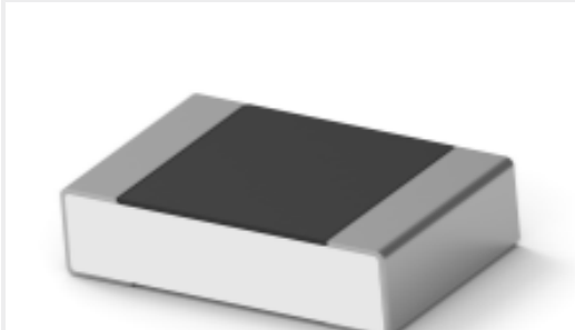
TE 产品编号4-2176373-3 RQ 0805 27R4 0.1% 10PPM 1K RL
