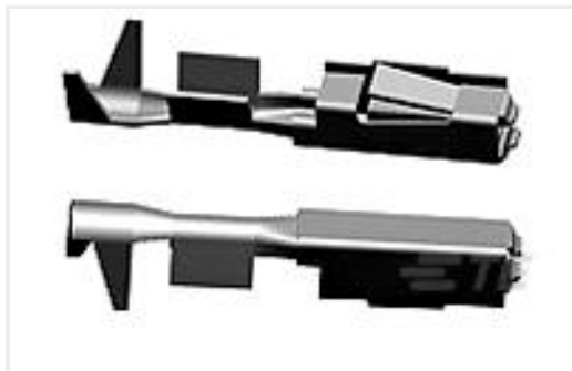
TE 产品编号5-1452013-1 MQS0,63 Au rec LL unseal. 0,5-0,75
