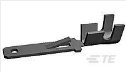
TE 产品编号160691-2 FF 250 TAB 22-18AWG TPBR
