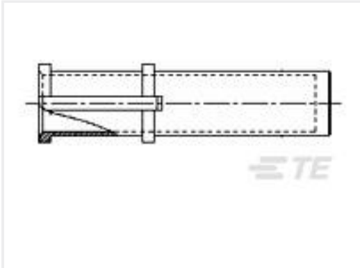
TE 产品编号688576-000 HEX07-AC
