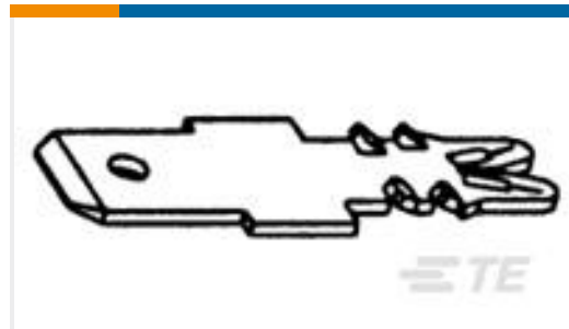
TE 产品编号4-1601011-1 031-023-000=TAB,187X020,STDSMZ
