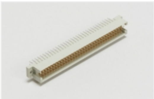
Eurocard 连接器(19)
