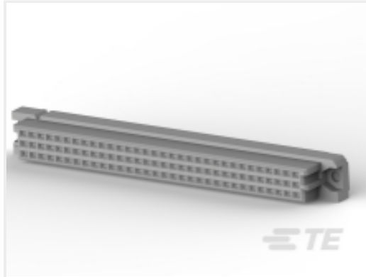
TE 产品编号 5535043-5 ASSY,RECEPTACLE,EUROCARD,TYPE
