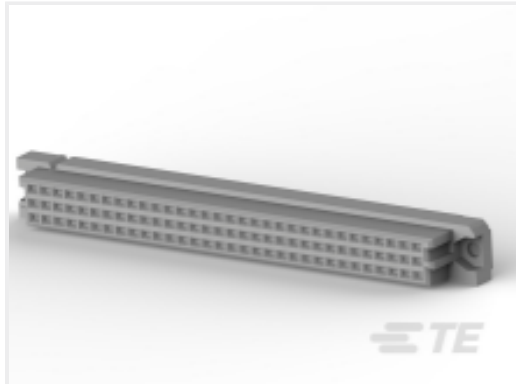
TE 产品编号 5535032-4 ASSY,RECEPTACLE,EUROCARD,TYPE C,LEAD-FREE,96 POS,19
