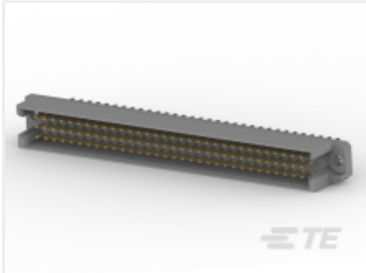
TE 产品编号 5650889-5 ASSY,PIN,EUROCARD,TYPE R,LEAD-FREE,96,19
