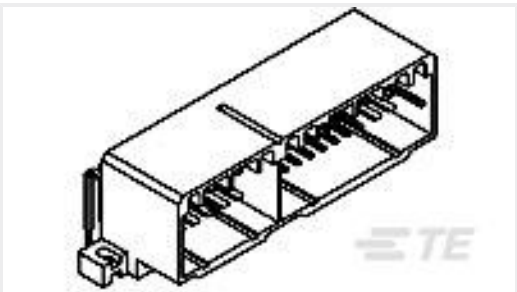
TE 产品编号173866-6 070 MULTILOCK CAP ASSY 30P
